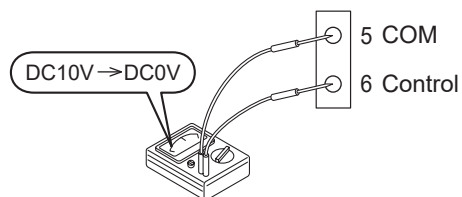
[Εικ. 9] Τάση της αναμεικτικής τριόδου (έλεγχος)
