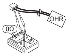
[Εικ. 6] Αντίσταση του ρελέ προστασίας υπερθέρμανσης του συμπιεστή
