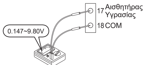
[Εικ. 7] Τάση του αισθητήρα υγρασίας
