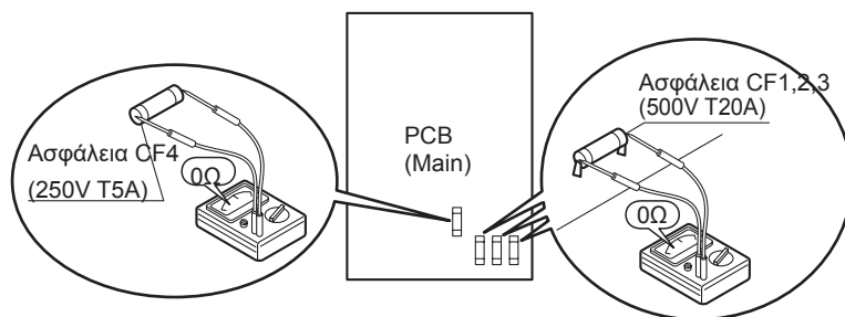
[Εικ. 1] Ηλεκτρική συνέχεια του ρεύματος της ασφάλειας της κεντρικής πλακέτας PCB (Main)
